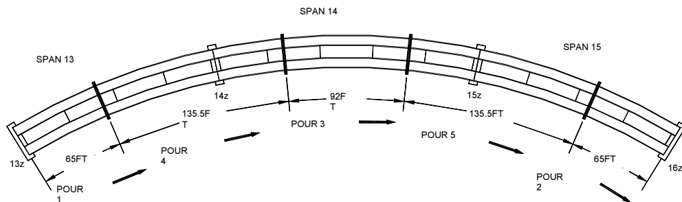
Figure 2.3: Concrete Pour Sequence
