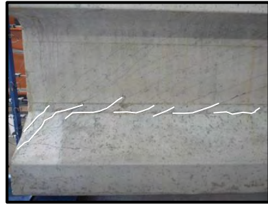
(D) Horizontal shear in Tx46
