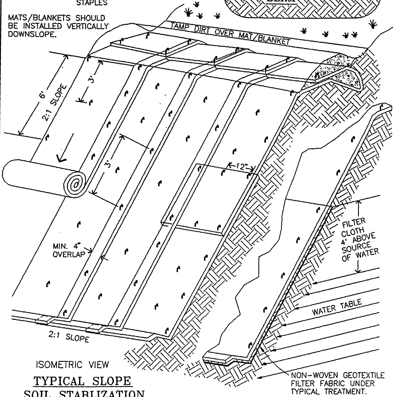
BERM
