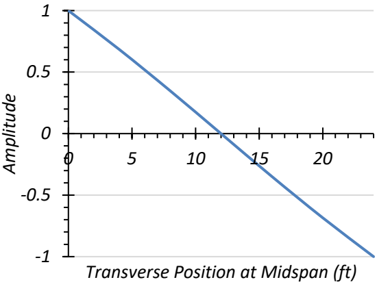
(b) Torsional Mode ( f=6.41 Hz)
